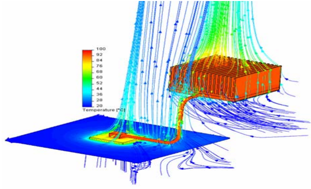
带热管散热器热分析
