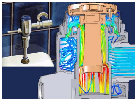
某水龙头内部流动分析(JOHNSON)
