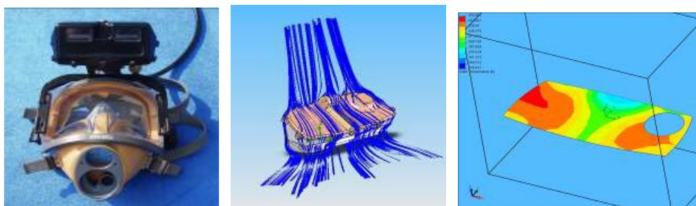
深水头盔目镜的温度场与压力场模拟 (Steam Machines Inc)
