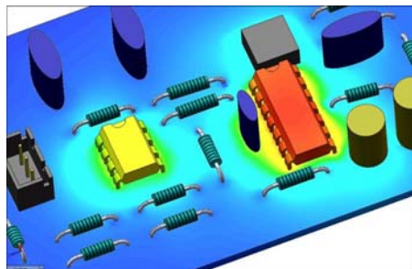
PCB 板及详细器件温度分布
