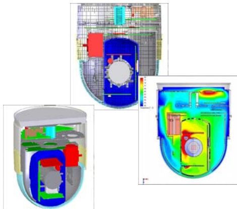
监控头热分析
