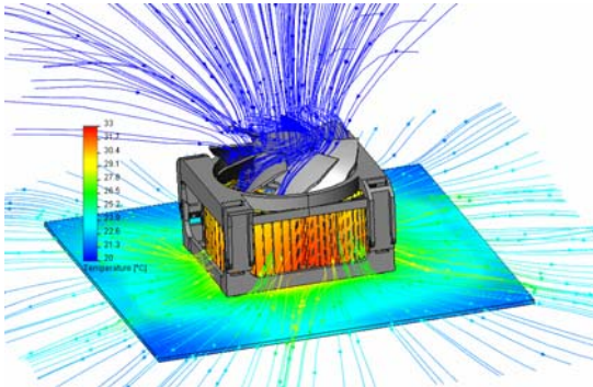
散热器流场流线及温度分布
