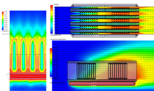
某空调换热器散热分析
