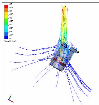
某高能灯辐射散热
