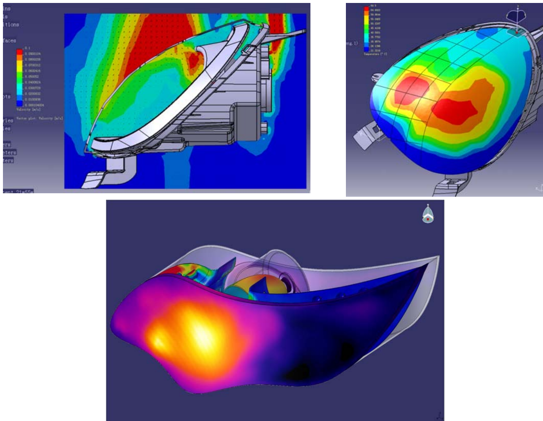
某车灯散热分析
