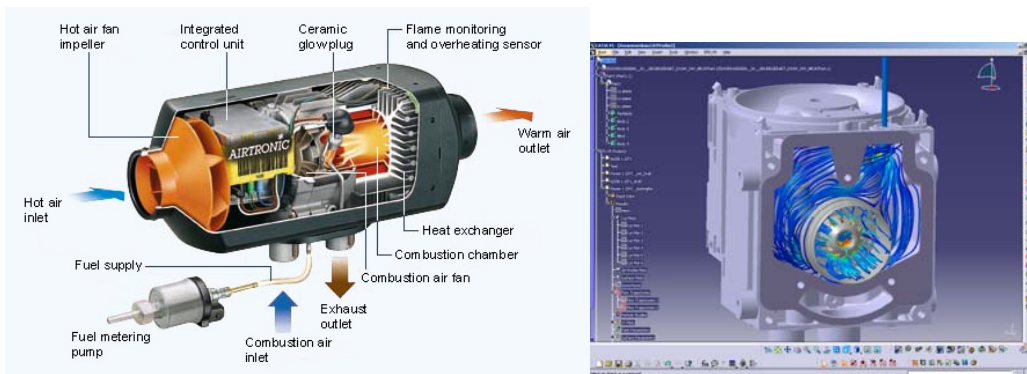
某车用空气加热器流动换热分析
