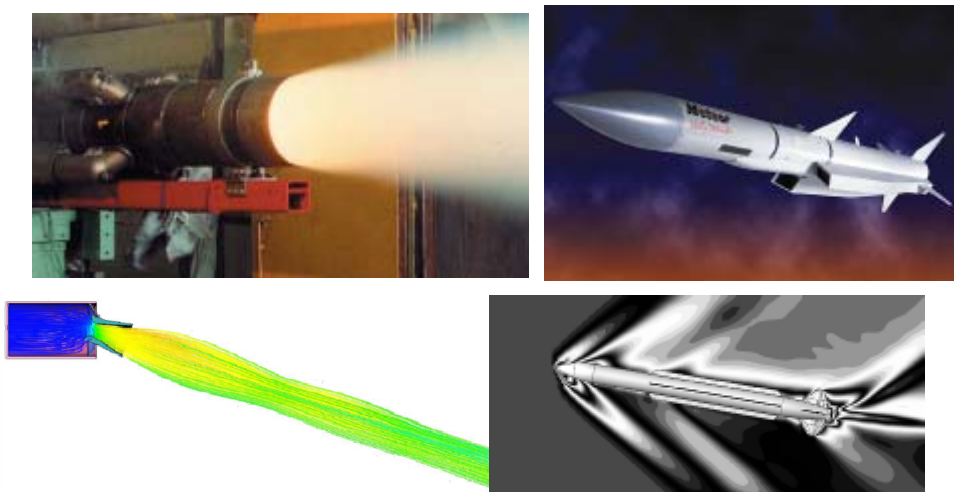
某导弹的推进仿真模拟 (Bayern-Chemie)
