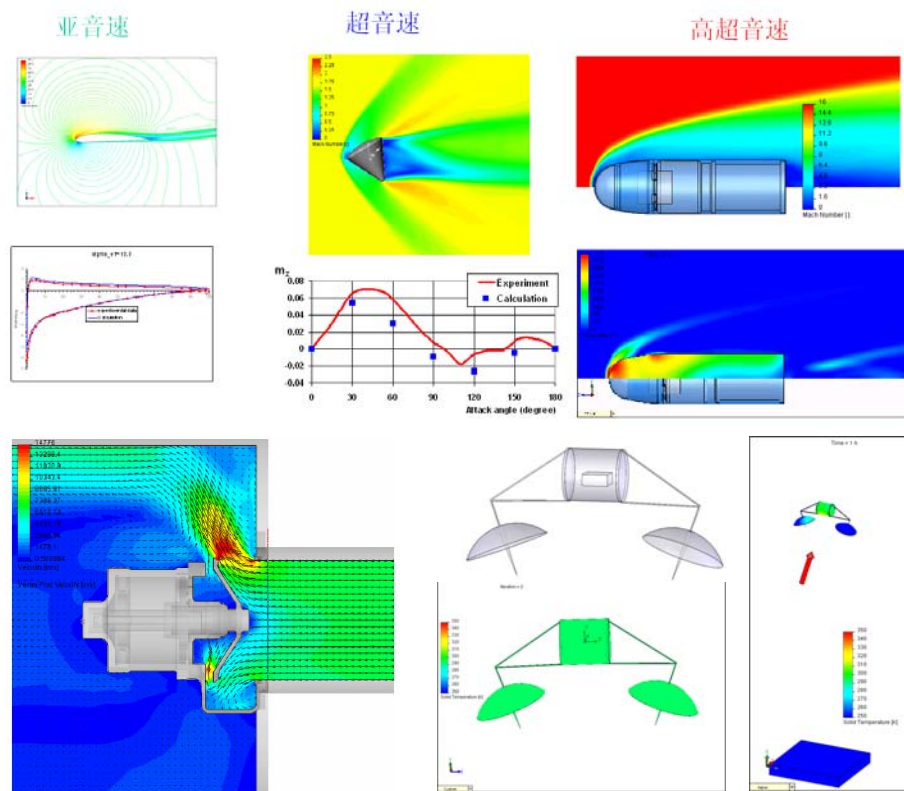
某航空航天用液轮机流场
