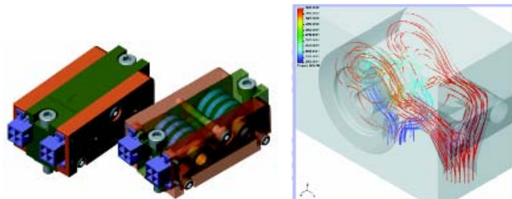
某高速阀门三维结构外形和内部流线图 (STURMAN INDUSTRIES)
