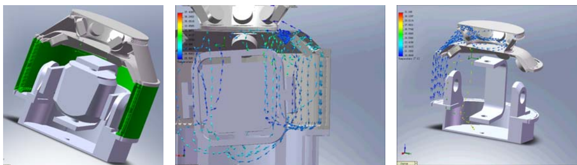
某导航陀螺系统温控
