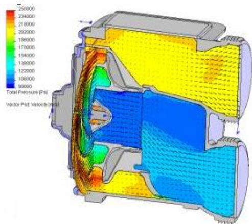
某离心泵压力分布、速度矢量图
